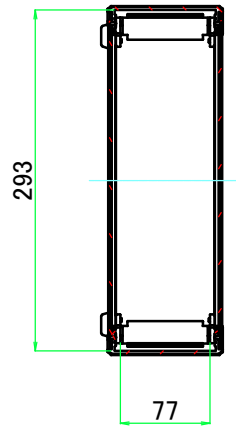
A-A ( 1 : 6.5 )
