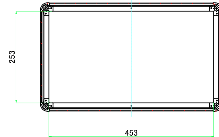
C-C ( 1 : 6.5 )
